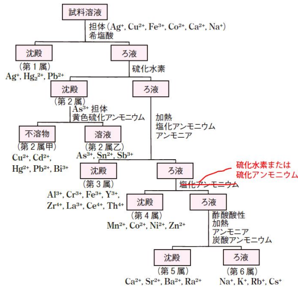
図 6.1 沈殿法による系統的分離
