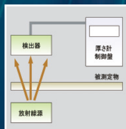
厚さ計(透過形)の原理
