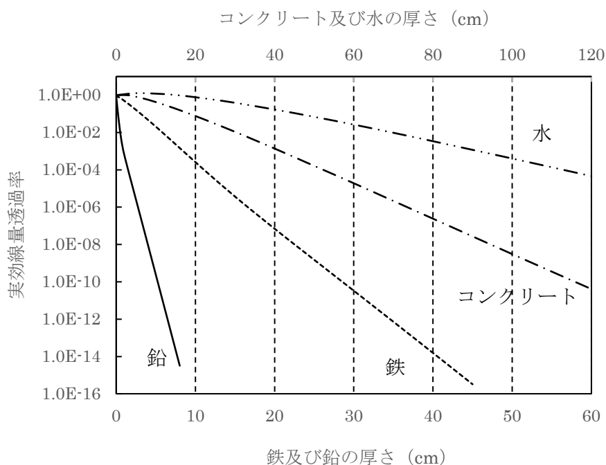
図 Lu-177 の実効線量透過率 F_a 2)
