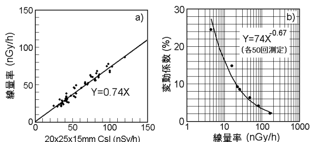
図4 線量計の校正 a) と変動係数 b)
