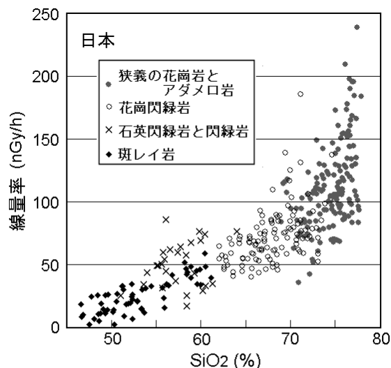
図2 日本における深成岩の岩石種と線量率
