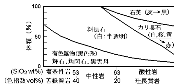
図 1 深成岩の鉱物組成
