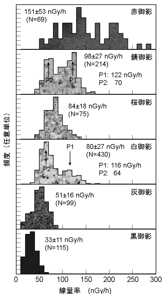
図6 御影石の線量率の頻度分布。Nは試料数
