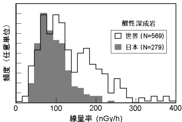
図3 日本と世界の酸性深成岩線量率
