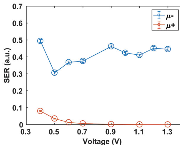
図3 ソフトエラー率 (SER; Soft error rate) 4)
