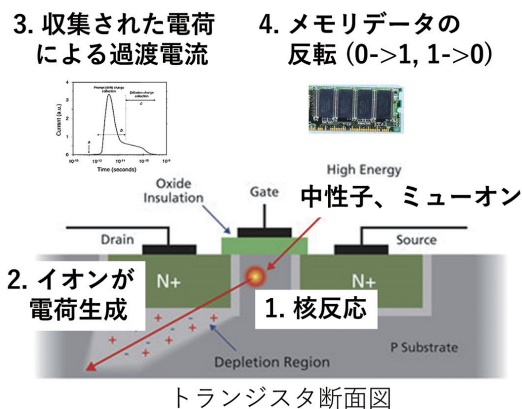
図 1 ソフトエラー
