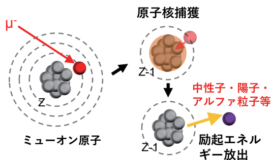
図 2 負ミュオン捕獲反応
